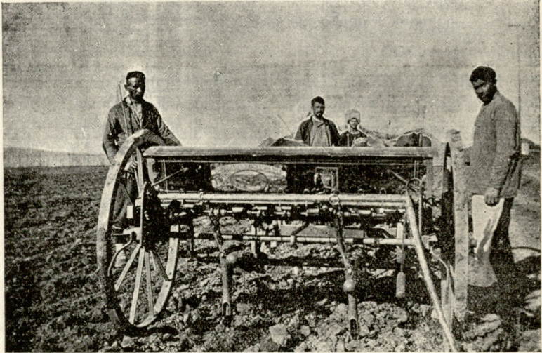
მწკრივად სათესი მანქანა ქართულ ს. სამ. საზოგ. მომზადებულია სიმინ- დის სათესად; ველის სიგანე 15¼ გოჯია. სოფ. ზემო-გომში (გორის მაზრა).
