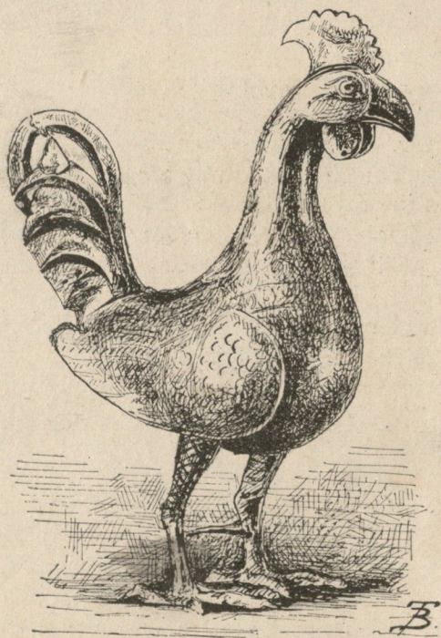
Coq en bronze, du Daghestan Collection du G-al de Péters. Dessin de Baerenstamm
