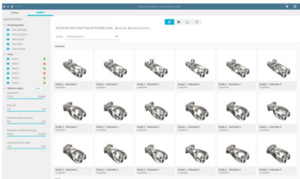
სურ. 5 რაკეტის ძრავის სამაგრის ფორმის სინთეზი
