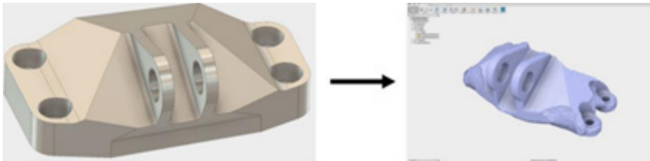
სურ. 4 რაკეტის ძრავის სამაგრის ტოპოლოგიური ოპტიმიზაცია
