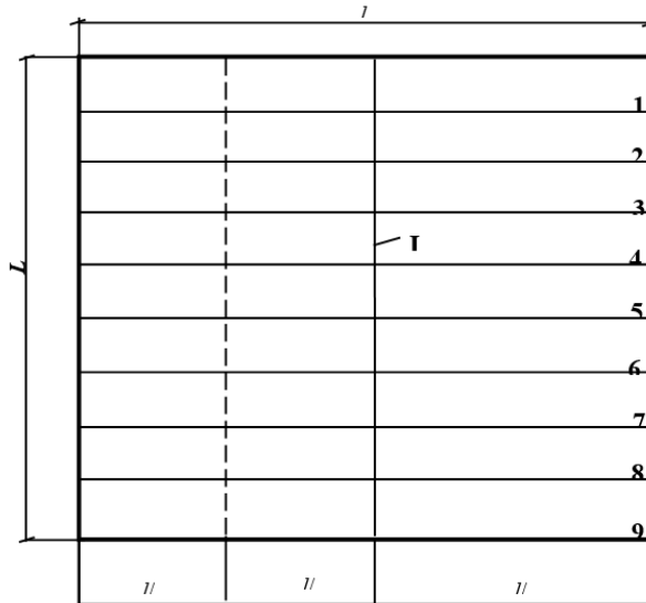
ნახ. 1. თვითმორთვის ოპტიმალური მანძილების დასადგენი სქემა – ორსაწევბაგირიანი განივგადასატანი საბაგრო დანადგარის გამოყენების დროს
