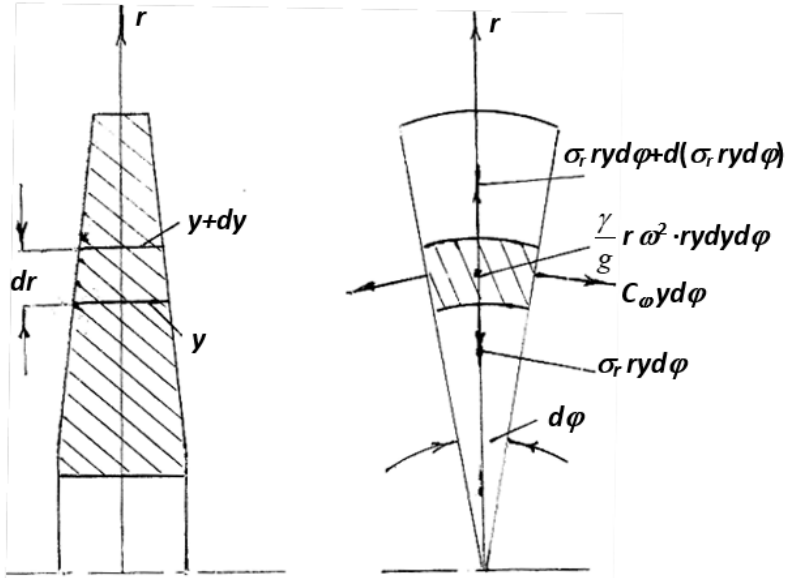
ნახ. 2. მბრუნავი დისკის ელემენტზე მოქმედი ძალები
