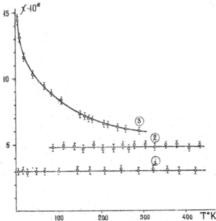
рис. 1. Температурная зависимость удельной восприимчивости соединений системы UMn_2 - UCo_2 . Кривая 1 соответствует соединению UCo_2 , и кривая 2 - соединению UMn_2 , кривая 3 - твердому раствору 50\% UMn_2 - 50\% UCo_2
