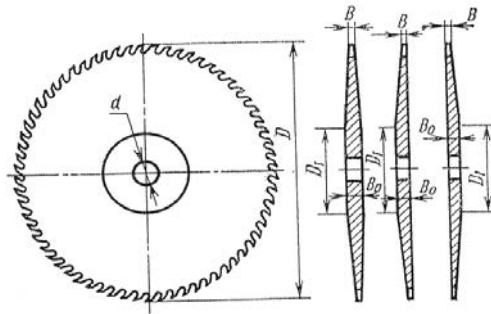
ნახ. 1. მრგვალი კონუსური ხერხი ა – ორმხრივი; ბ – მარცხნივ კონუსური, გ – მარჯვნივ კონუსური.
