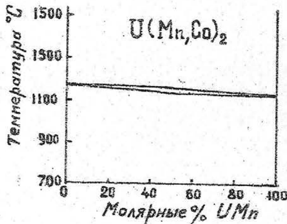
Рис. 2. Диаграмма состояния сплава (UM_nCo)_2
