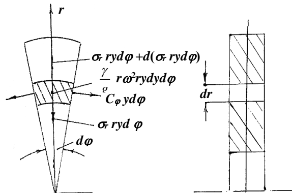
ნახ. 2. მბრუნავი დისკის ელემენტზე მოქმედი ძალები
