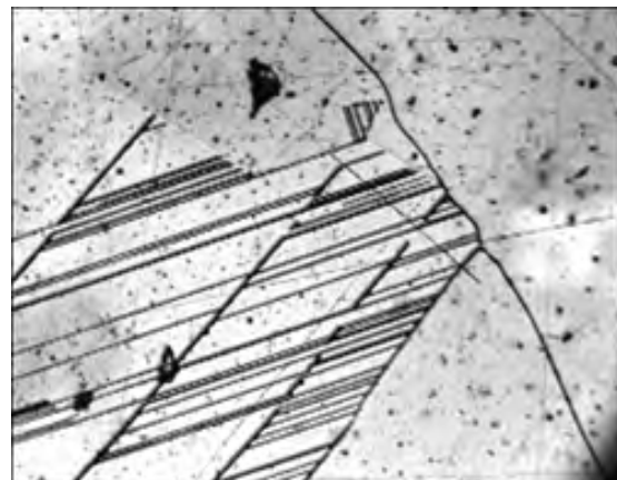
ნახ. 1. ფოსფორით ლეგირებული Si და Si 0.98 Ge 0.02 შენადნობის მიკროსტრუქტურა
