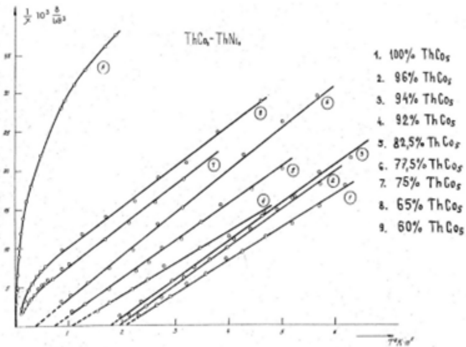
ნახ. 5. კუთრი ამთვისებლობის ააორატულ ტემპერატურაზე ( T^2 ) დამოკიდებულება ThCo_5 - ThNi_5 მყარი ხსნარების სისტემისთვის
