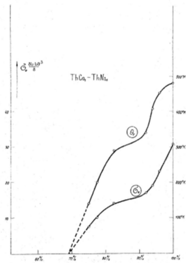
ნახ. 6. კიურის \theta_F ფერომაგნიტური ტემპერატურის დამოკიდებულება კუთრი სპონტანური დამაგნიტების სიდიდეზე \text{ThCo}_5 - \text{ThNi}_5 მყარი ხსნარების სისტემისთვის
