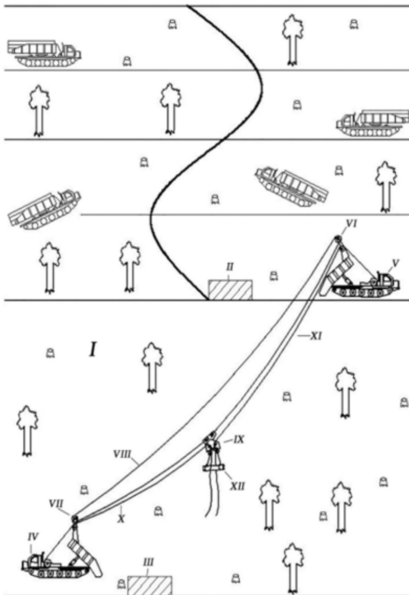
ნახ . 1 ტყეკაფების ათვისებისა და ცივაბო ფერდობების ტყით განახლების სამუშაო პროცესების კომპლექსური მექანიზაციის N 14 ტექნოლოგიური სქემა
