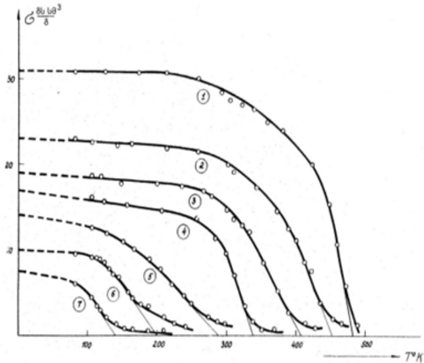
ნახ. 7. კუთრი დამაგნიტების დამოკიდებულება ტემპერატურაზე ThCo_5 - ThNi_5 ნაერთებში
