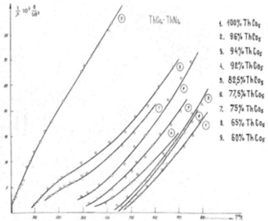
ნახ. 4. კუთრი ამთვისებლობის ტემპერატურაზე დამოკიდებულება ThCo_5 - ThNi_5 მყარი ხსნარების სისტემისთვის
