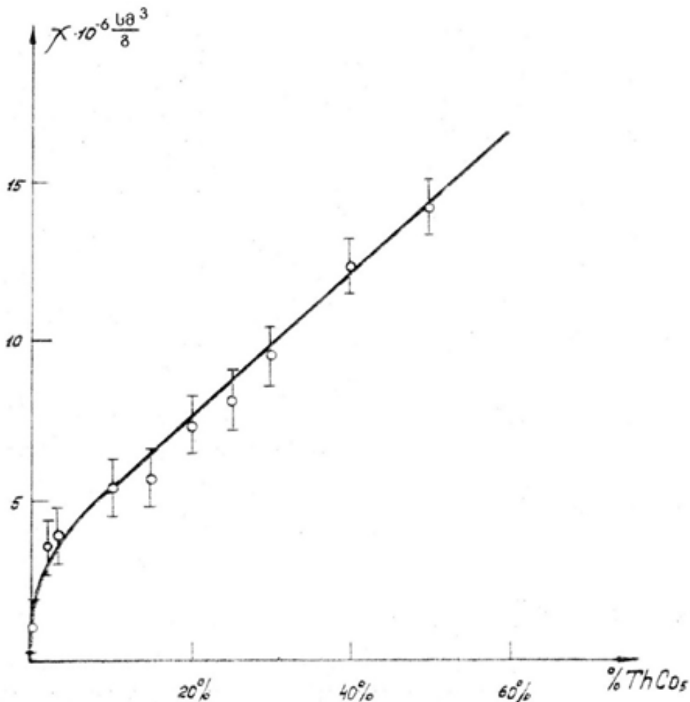
ნახ. 3. ტემპერატურაზე დამოუკიდებელი კუთრი ამთვისებლობის დამოკიდებულება ThCo 5 – ThNi 5 მყარი ხსნარების შემადგენლობაზე
