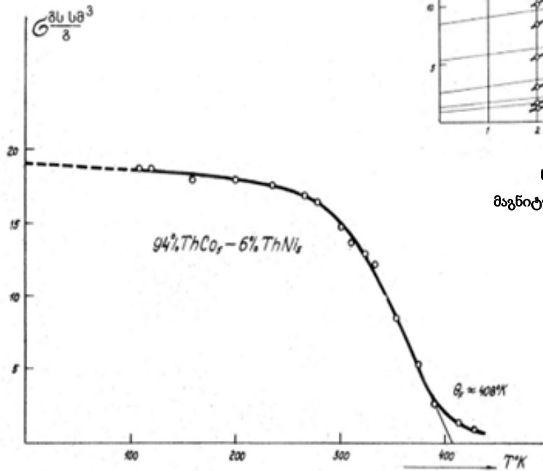
ნახ. 2. კუთრი სპონტანური დამაგნიტების დამოკიდებულება ტემპერატურაზე, 94% ThCo_5 - 6% ThNi_5 მყარ ნაერთში
