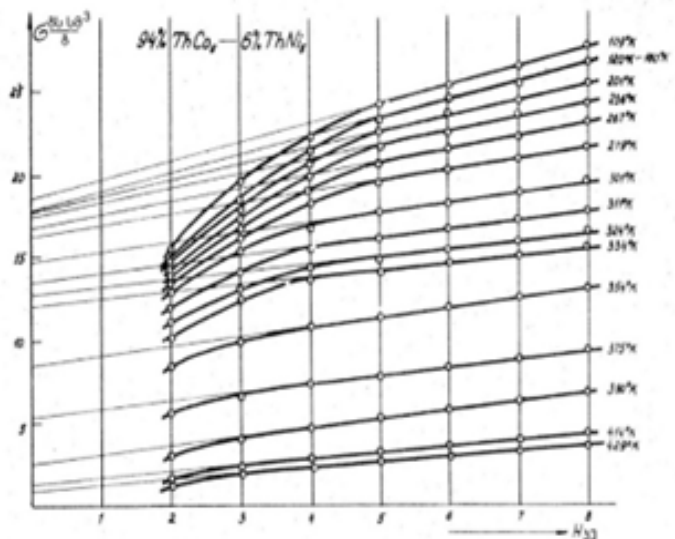
ნახ. 1. კუთრი დამაგნიტების თანაობის დამოკიდებულება მაგნიტურ ველზე 94% ThCo_5 - 6% ThNi_5 მყარი ნაერთებისთვის
