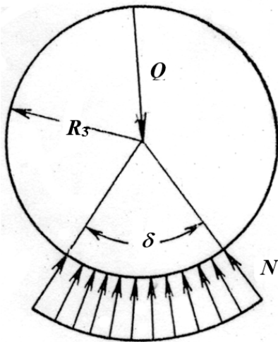
ნახ. 2. დასამუშავებელ დეტალზე მოქმედი წნევების გრაფიკი
