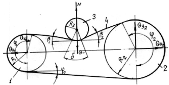
ნახ. 3. მრუდწირული დეტალების დასამუშავებელი ლენტური სახეხი ჩარხის საანგარიშო სქემა
