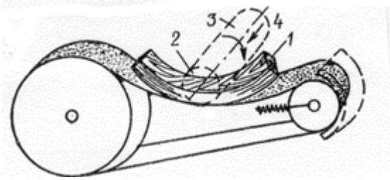
ნახ. 1. მრუდწირული დეტალების დასამუშავებელი ლენტური სახეხი ჩარხი
