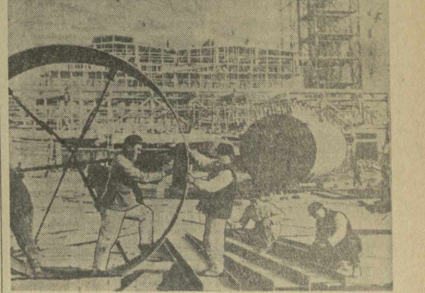
Китайская Народная Республика. На строительство химического завода в городе Ляньюэ — растущем индустриальном центре Северо-западного Китая. Фото Ся Ма. (Агентство Синьхуа).
